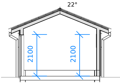
Snitt A-A
