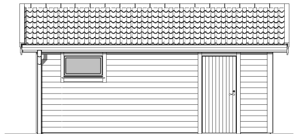
Fasade 4
